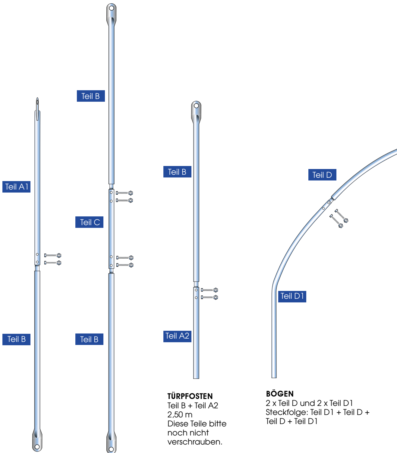
WINDVERBAND Teil A1 + Teil B 3,00 m
